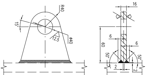
零件1-1详图 PIECE NUMBER 1-1 DETAILED DRAWING 不标注比例 SCALE
