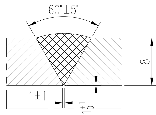
A,B类对接接头详图
