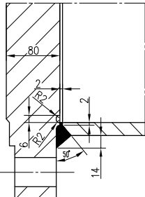
管板与筒体连接详图
